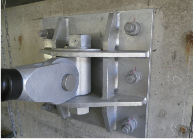
落橋防止ブラケット
