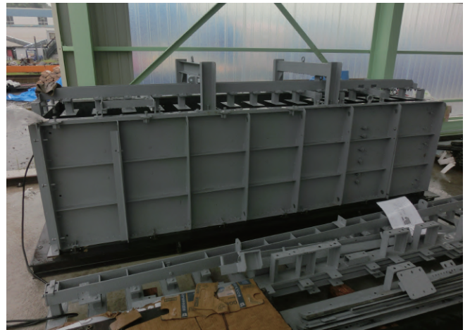
柱型枠
